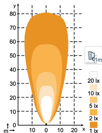
N73012 600 lm Flood TT DS - T987-102B
