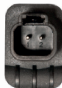
Built-in Deutsch DT-2 (2-pin)
